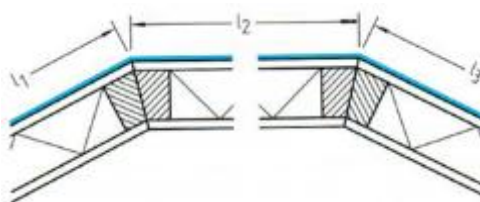
Figure 25: plus grande longueur développée l = l_1 + l_2 + l_3
