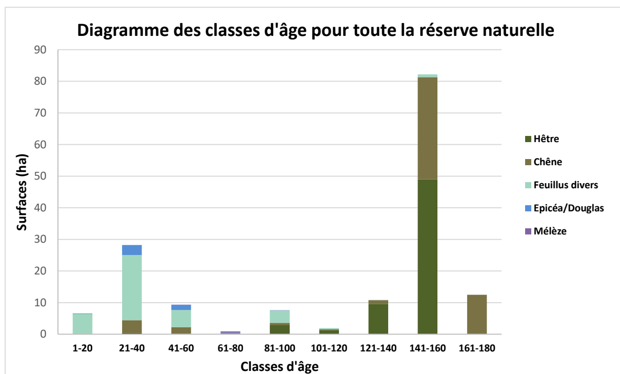
Fig. : 3-1 : Diagramme des classes d'âge pour toute la réserve naturelle (159,17 ha)
